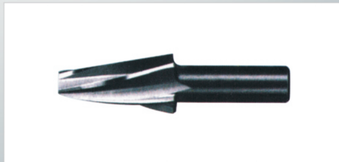
整體螺旋錐度鉸刀
